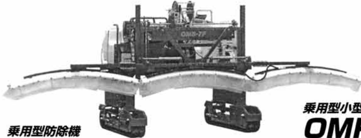
軌間幅1600~1850mm
