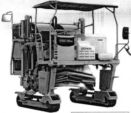
乗用型摘採機 OHC-8VB・10VB・20VB・30VB型 軌間幅1600~1850mm
